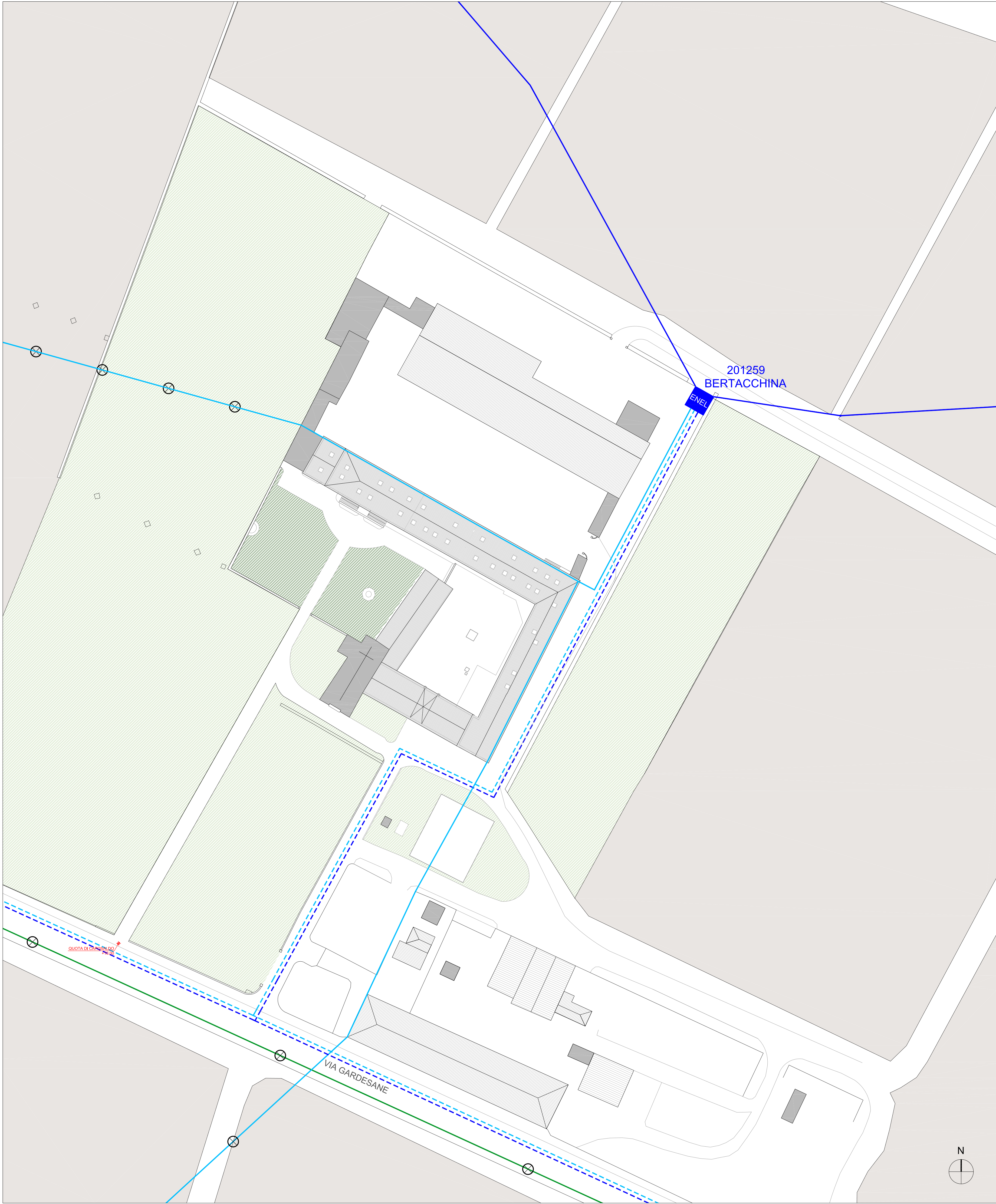
TAV. 1: RETE ELETTRICA E ILLUMINAZIONE PUBBLICA
